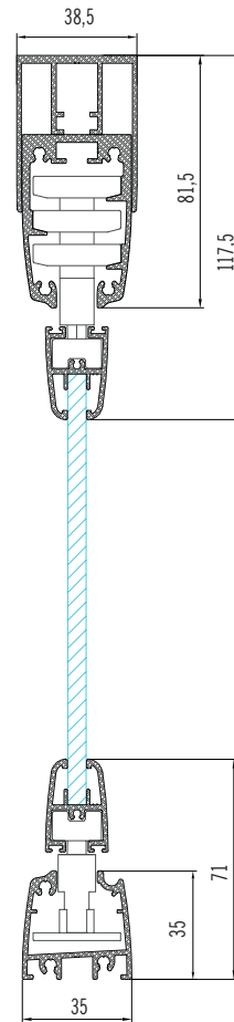
Perfil guía inferior Basic Pro
