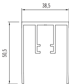
Perfil hoja 6mm Basic Pro
