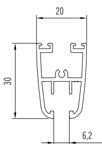
Perfil hoja 6mm Basic Pro
