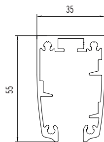
Perfil hoja 8mm Basic Pro
