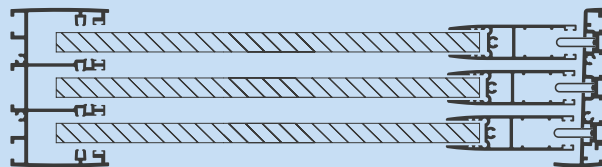
Vista sección paneles
