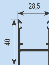
Perfil marco lateral
