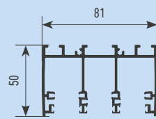
Perfil guía superior T3
